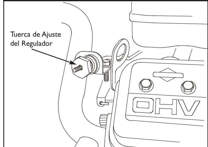
Figura 28 — Tuerca de Ajuste del Regulador
